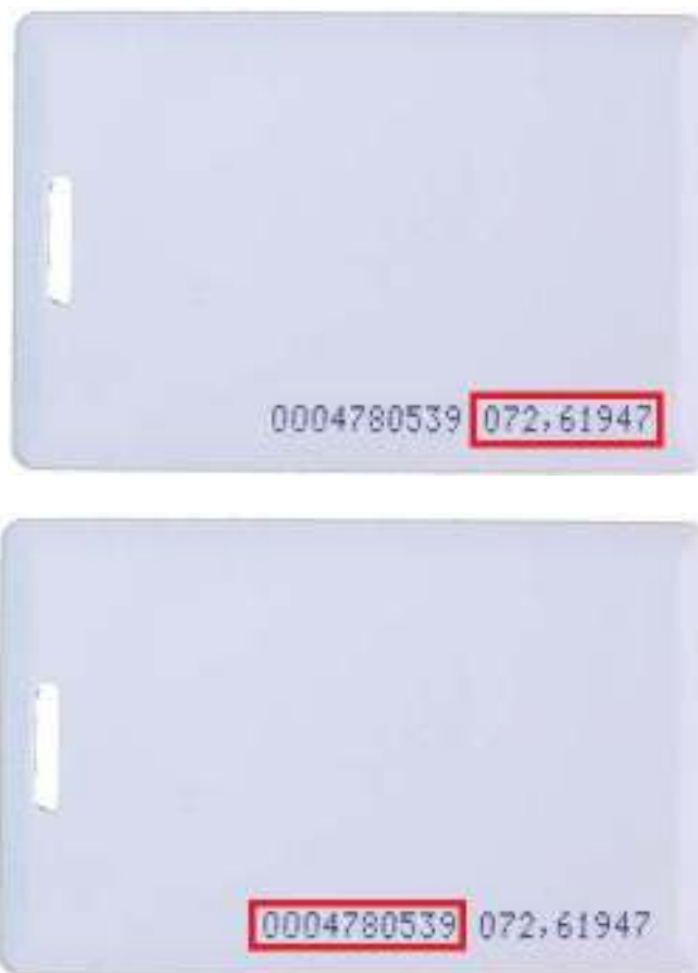
Рисунок 134. Карта EM Marine с различными вариантами записи её номера.
