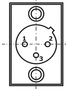
Рисунок 4 – Назначение контактов разъемов блока управления
