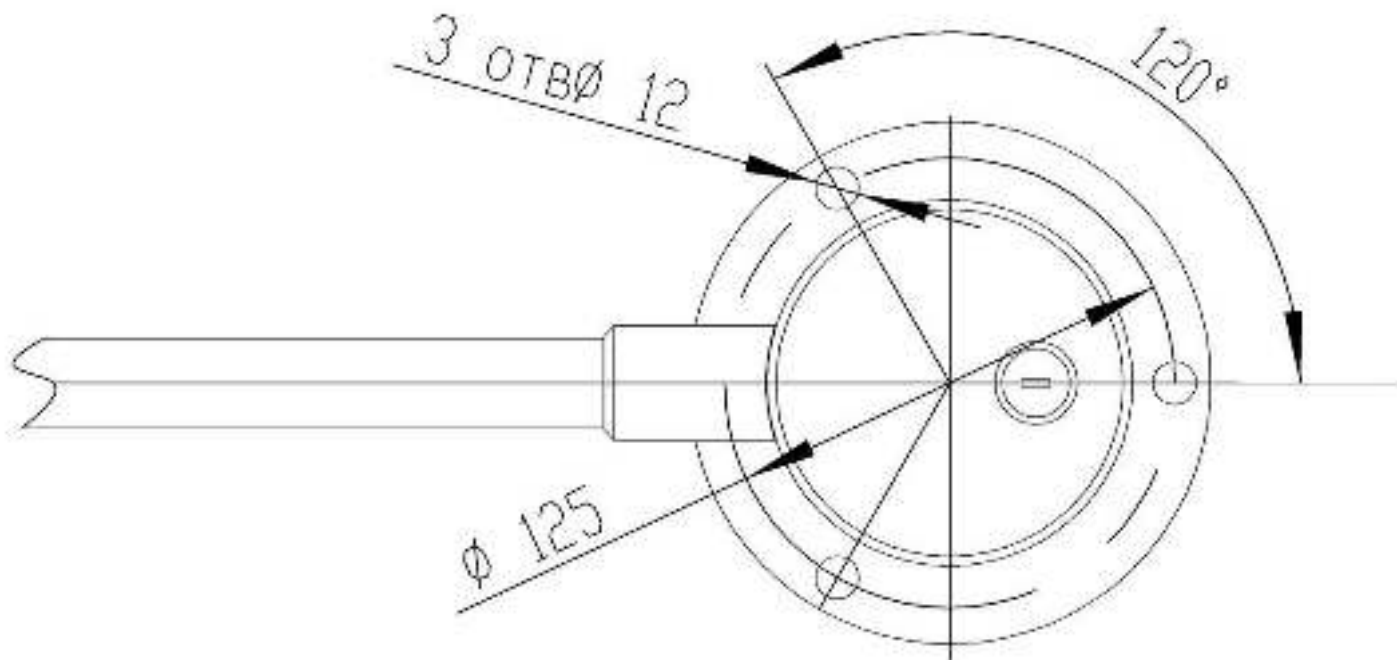
Рисунок 5 – Схема разметки для монтажа калитки
