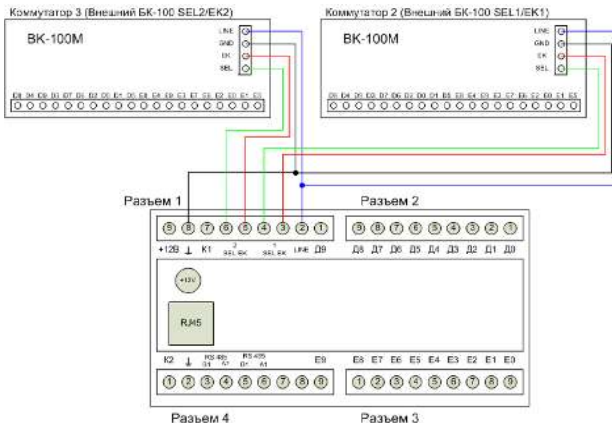
Рисунок 2. Схема подключения внешних БК-100 к ТИ-IPCS300.
