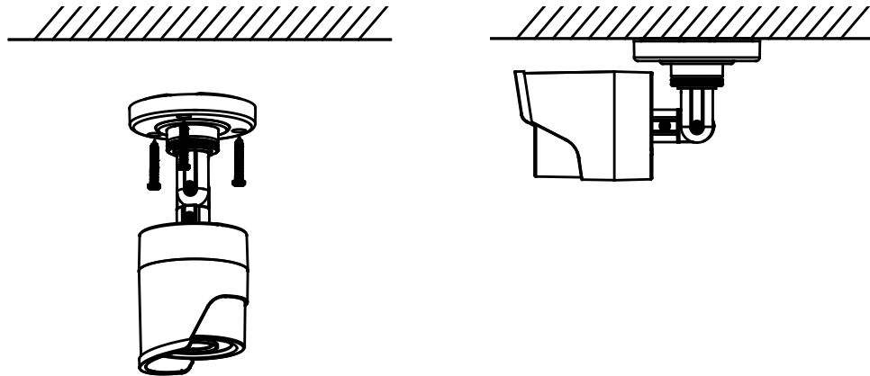
Рис.2.4.1.1 Установка видеокамеры LTV CTB-610
