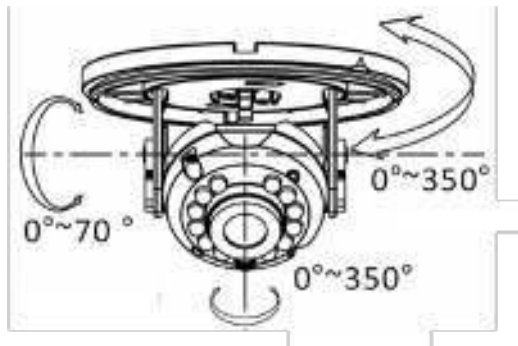
Рис. 4.4.1.3. Настройка позиционирования видеокамеры LTV CTB-710
