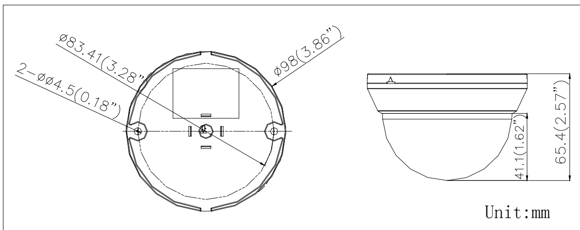
Рис. 4.2.1. Габаритные размеры видеокамеры LTV CTB-710
