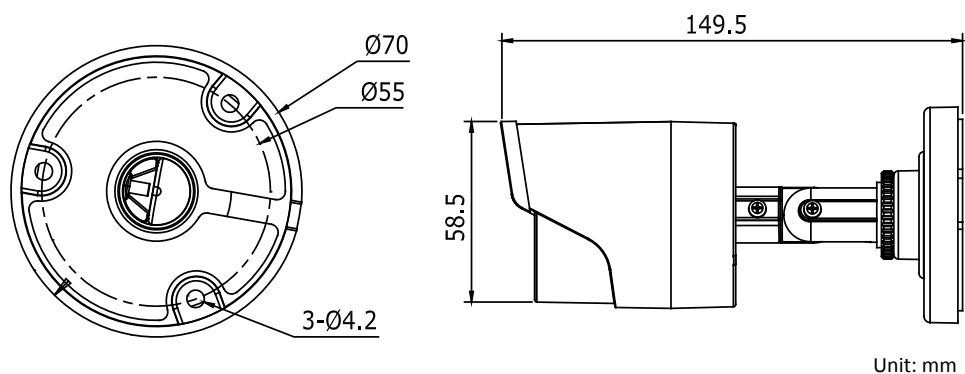
Рис.2.2.1. Габариты LTV CTB-610
