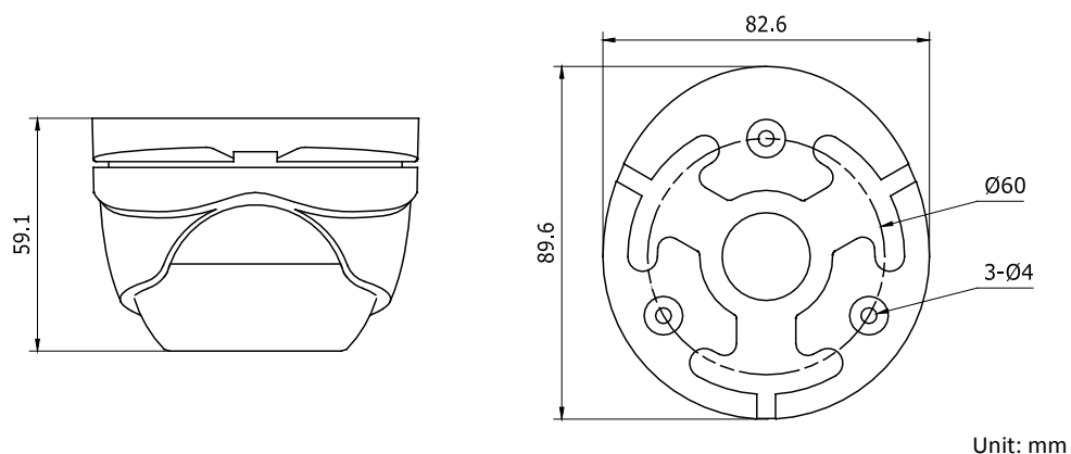
Рис. 3.2.1. Габариты LTV CTB-910
