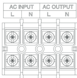
Клеммный блок
