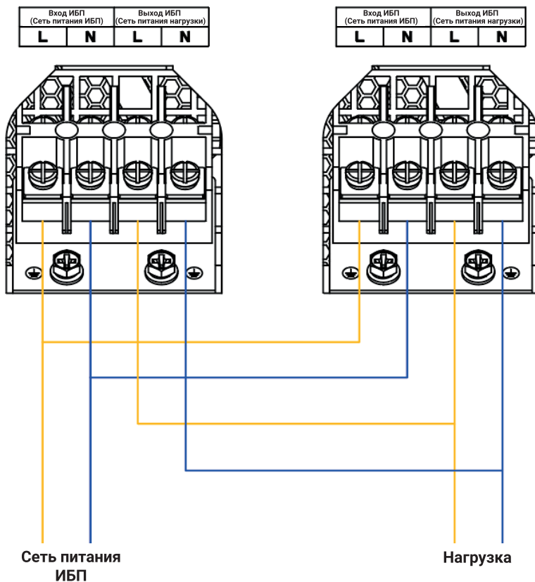
Подключение переменного тока к нагрузке
