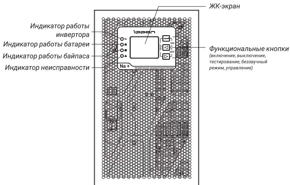
ИБП Na+ TA 6K / Na+ TA 10K
