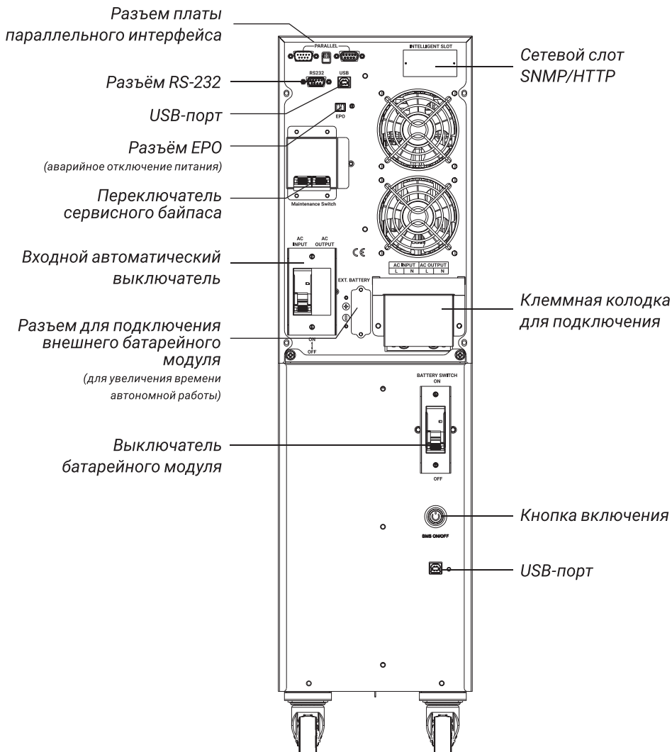
ИБП Na+ TA 6K / Na+ TA 10K
