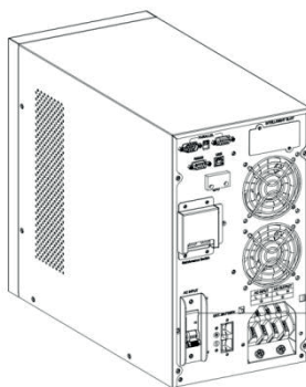
Входной автоматический выключатель
