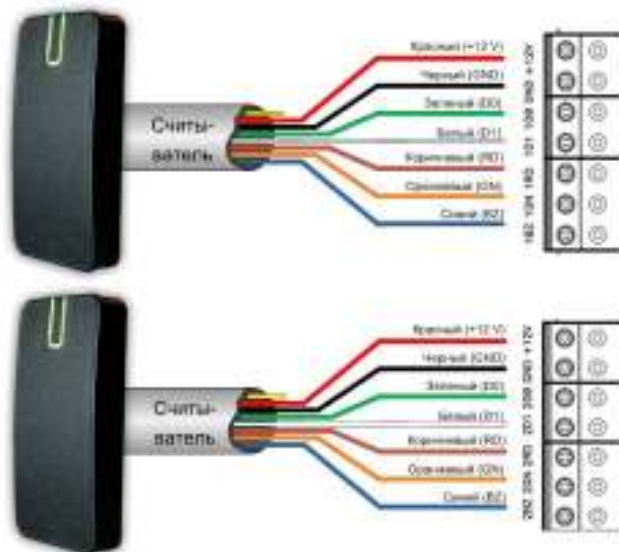
Рис.11. Подключение считывателей
