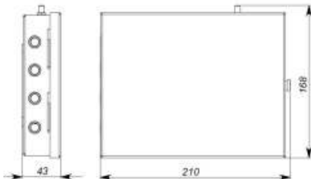
Рис 9. Габаритные размеры
