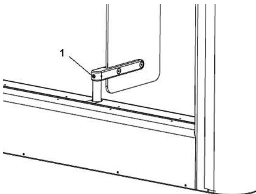
1 - стопорный винт
