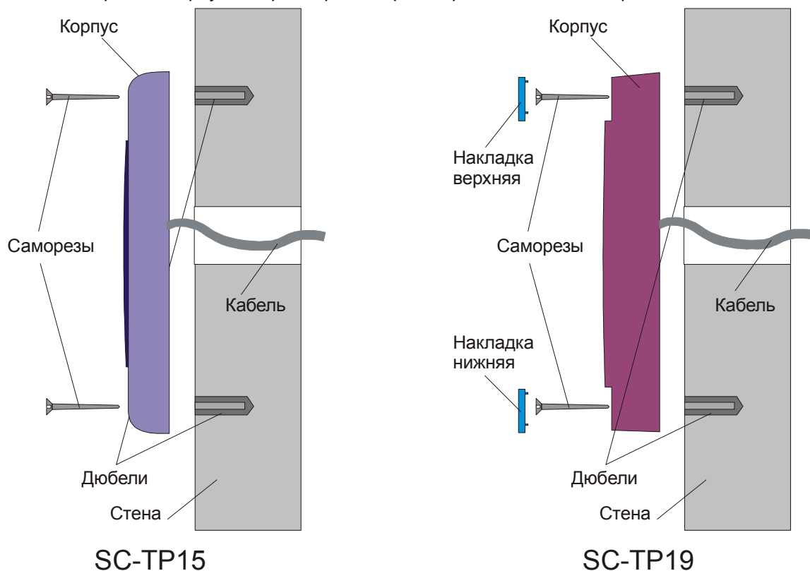
Рисунок 1. Крепление контроллеров.
