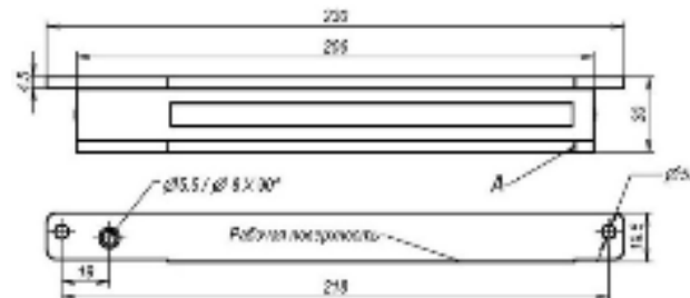
Рисунок 2 - Корпус
