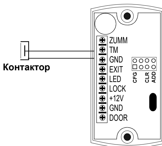
Рис.6 Подключение контактора
