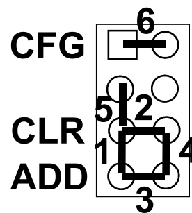
Рис.7 Перемычка
