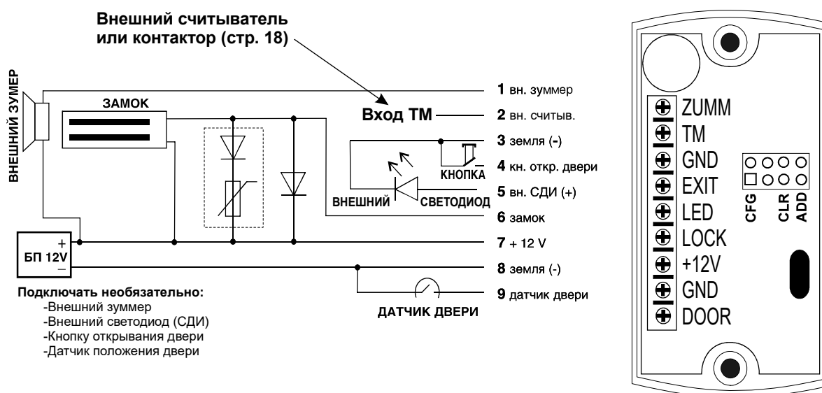
Рис. 3 Подключение внешних устройств
