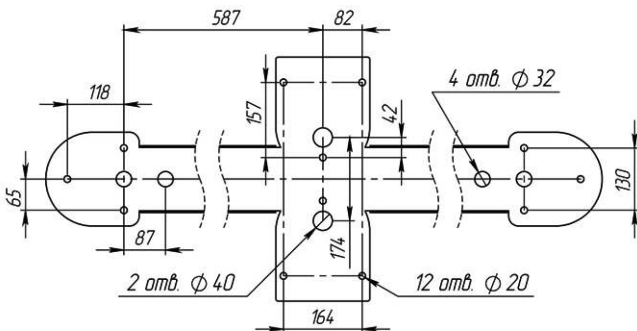
Рисунок 4 – Установочные размеры площадки турникета
