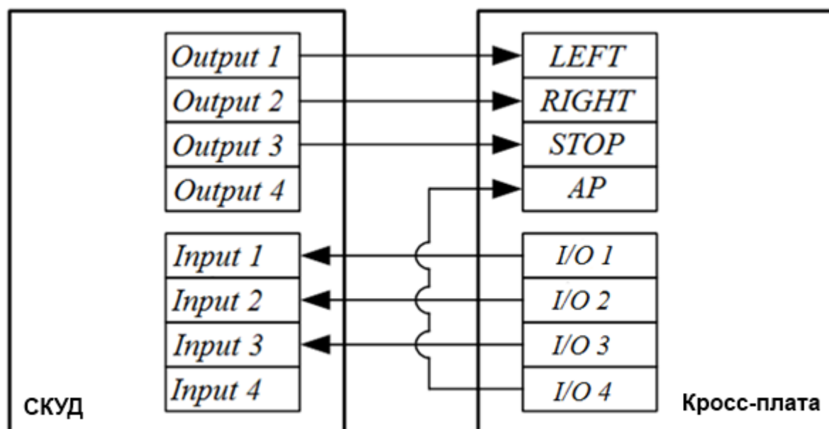
Рисунок 12 – Схема подключения ПУ к контроллеру СКУД
