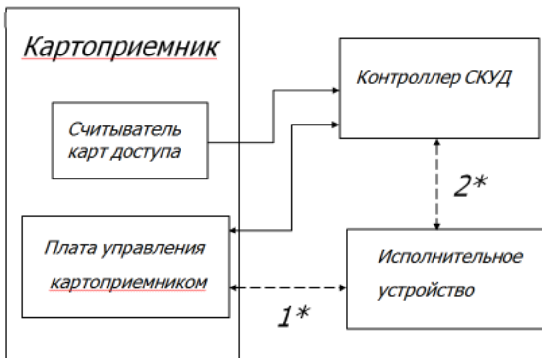
Рисунок 21 – Структурная схема №3
