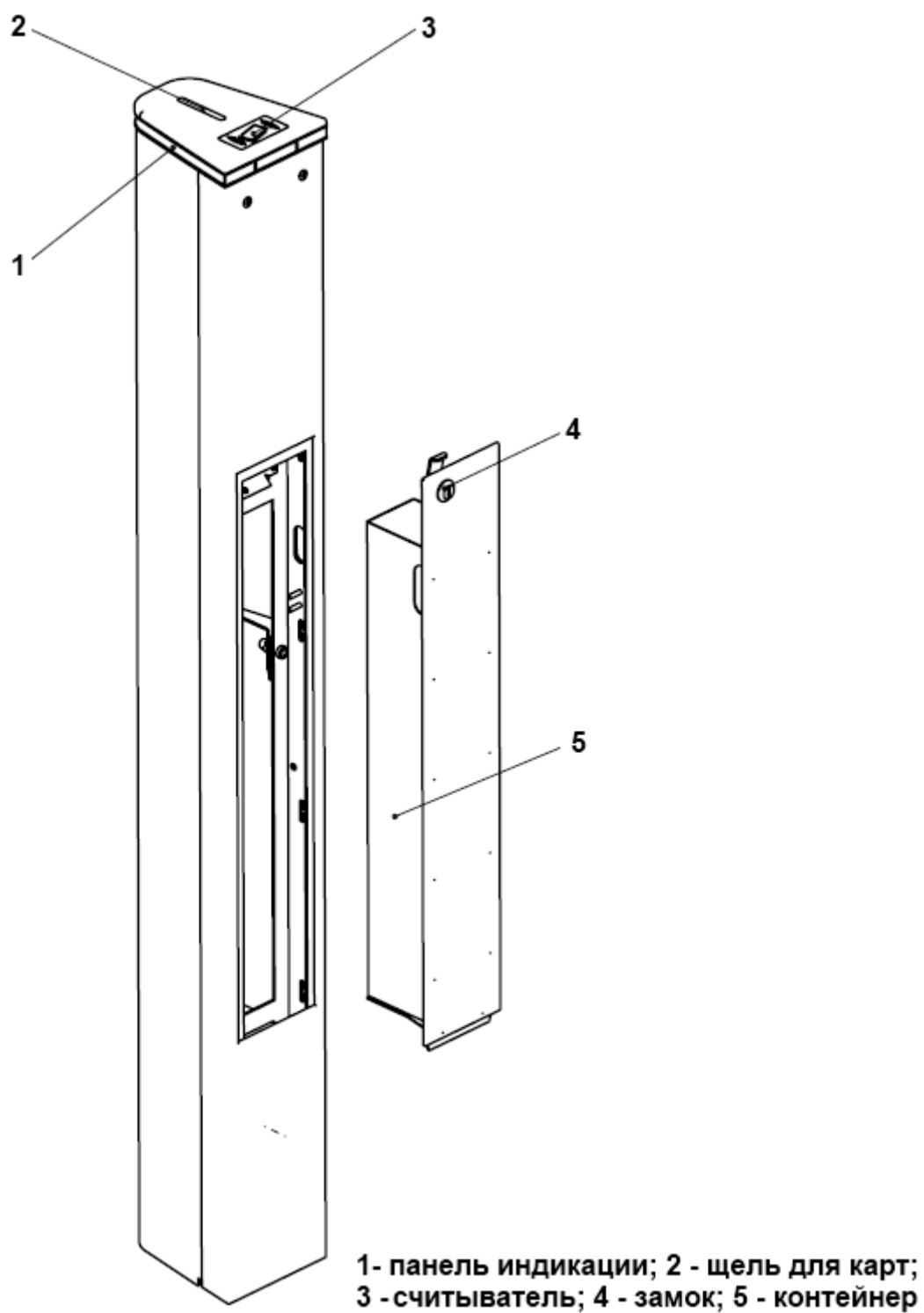
Рисунок 3 – Устройство изделия
