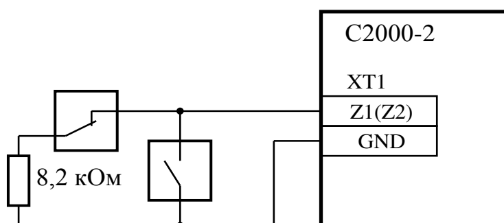
Рисунок 6 Схема подключения "нормально-замкнутых" и "нормально-разомкнутых" охранных извещателей, а также цепей разрешения считывания и открытия доступа в ШС1 и ШС2 контроллера "C2000-2"
