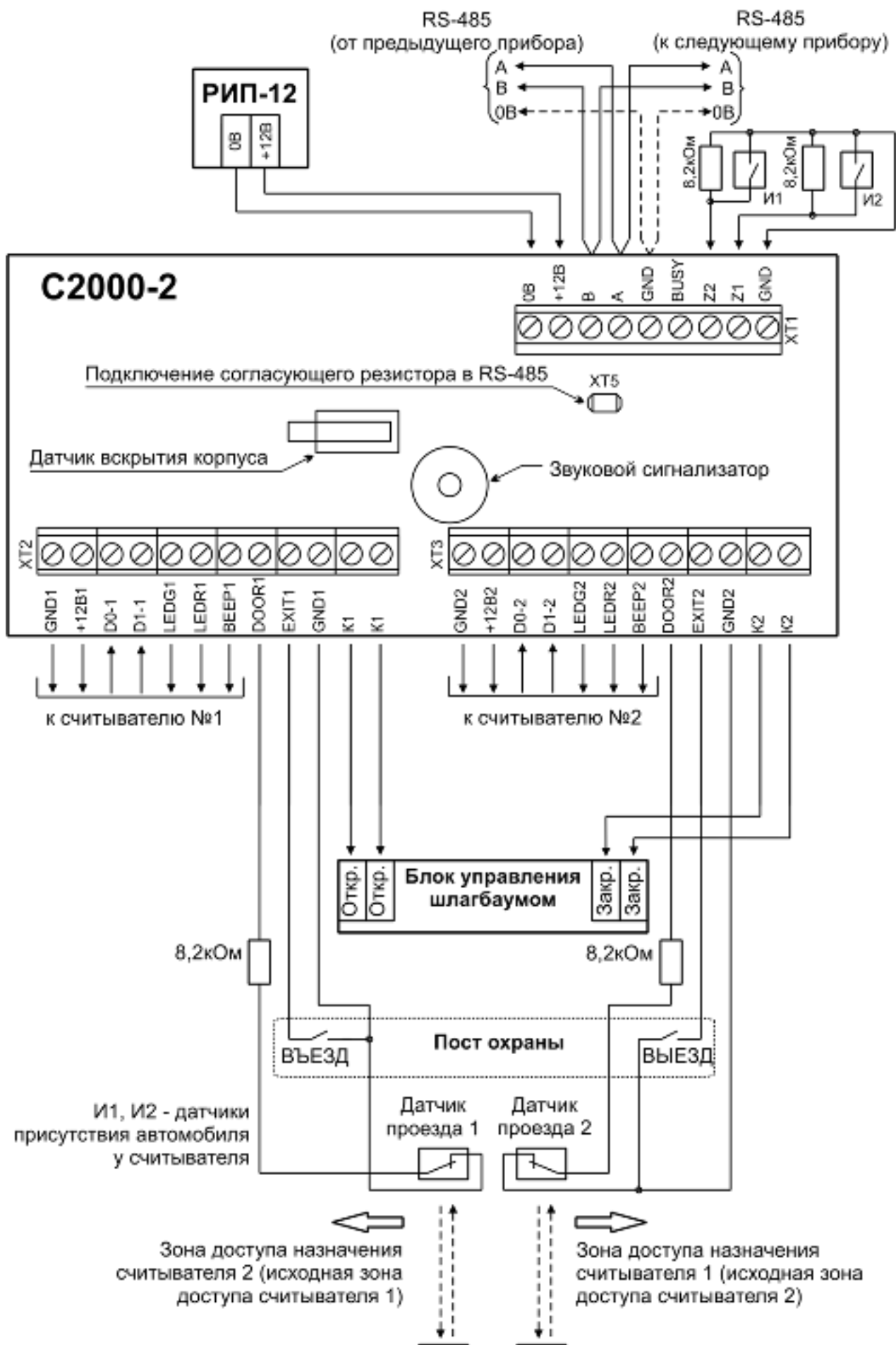
Рисунок 13 Схема подключения контроллера "C2000-2" в режиме "Шлагбаум"
