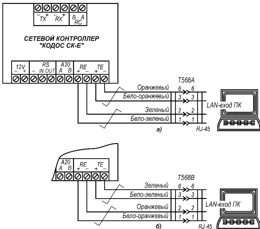
Рис. 7.1. Схема подключения сетевого контроллера к ПК:
