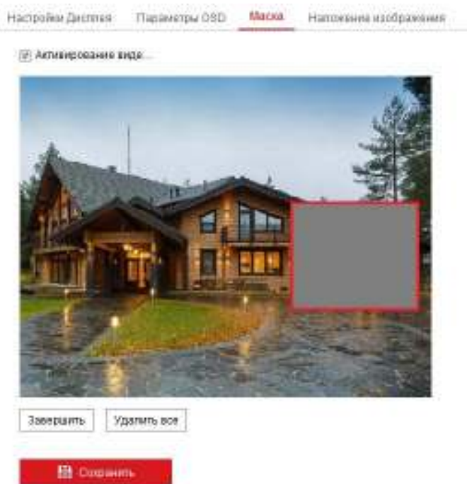
Рисунок 9-7 Настройки маски
