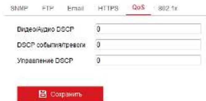
Рисунок 7-15 Настройка QoS
