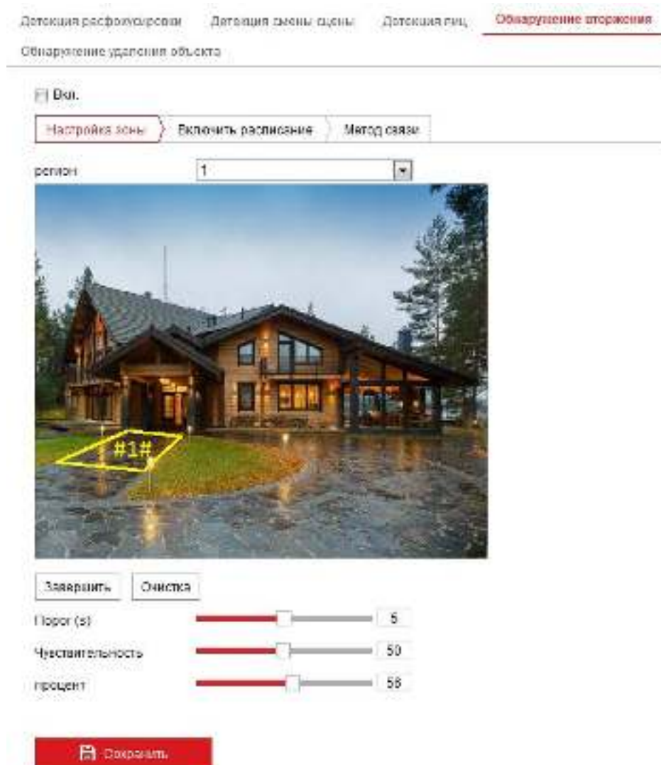
Рисунок 10-20 Обнаружение вторжений
