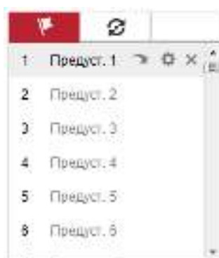
Рисунок 5-4 Установка предустановки
