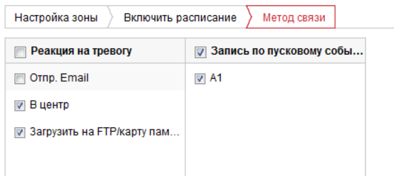
Рисунок 10-4 Методы связи
