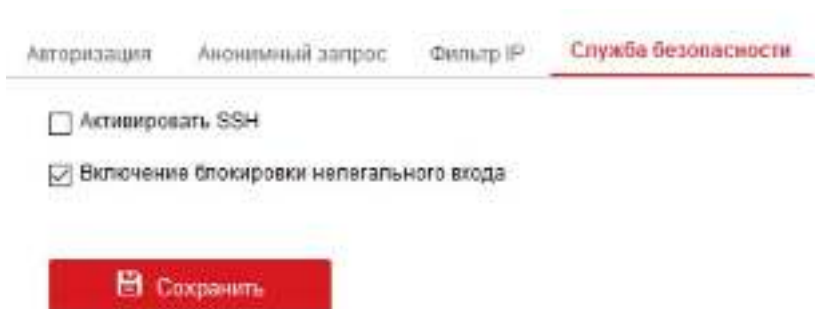
Рисунок 6-19 Служба безопасности
