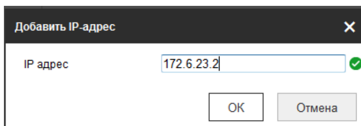
Рисунок 6-17 Добавление IP-адреса
