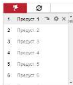
Рисунок 5-5 Вызов предустановки
