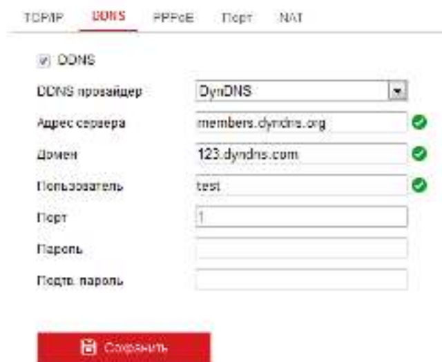
Рисунок 7-2 Настройка DynDNS
