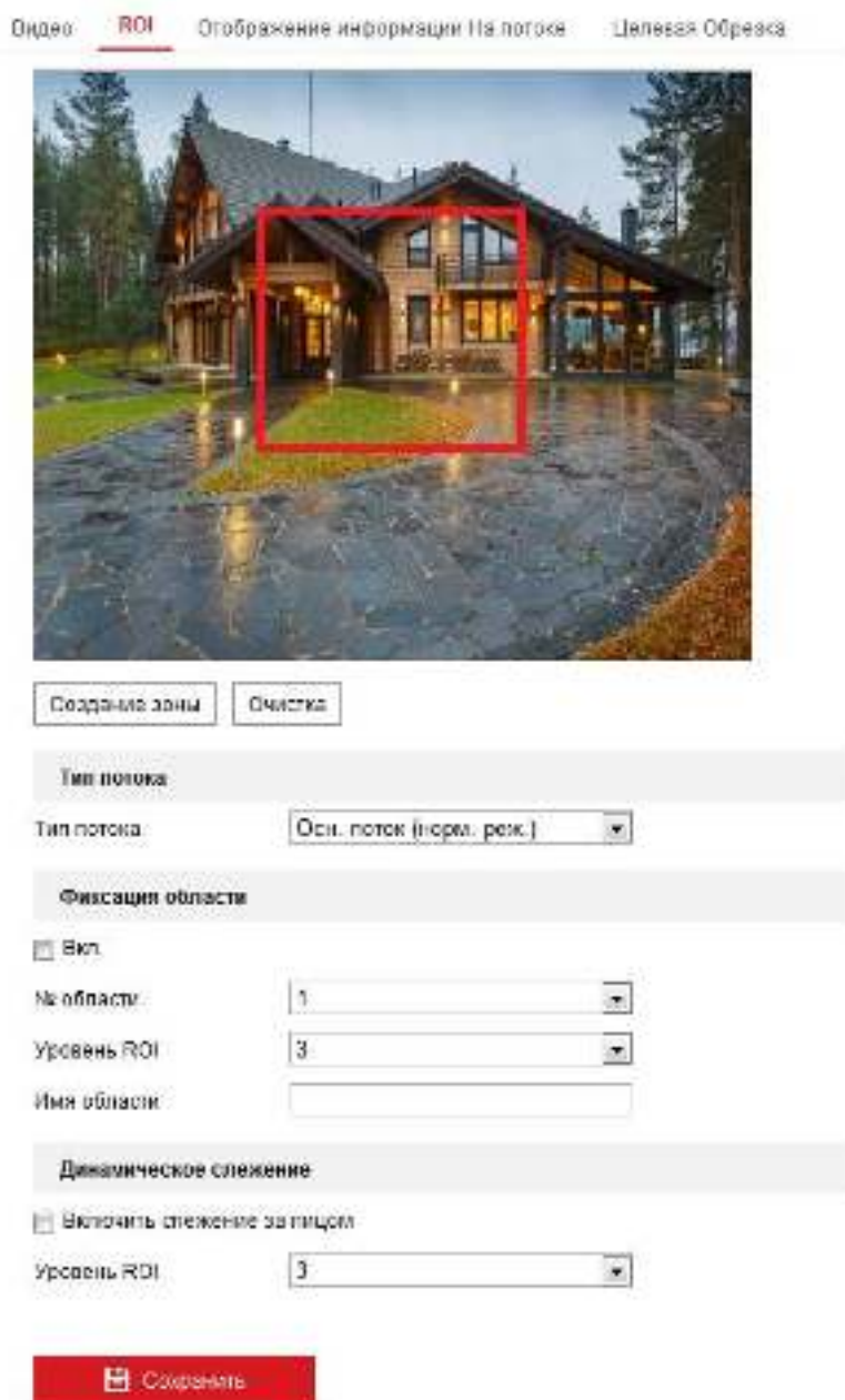
Рисунок 8-3 Настройка ROI
