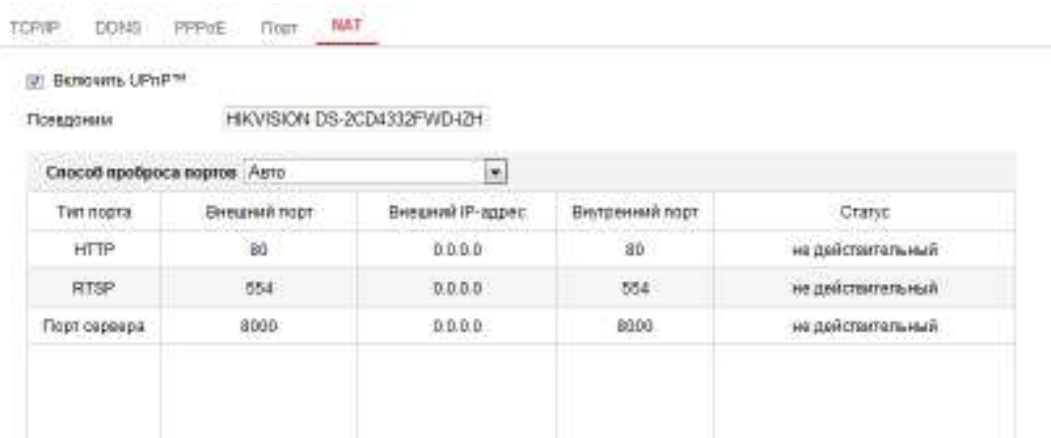
Рисунок 7-8 Настройка NAT
