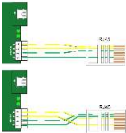
Рис.20. Подключение кабеля Ethernet
