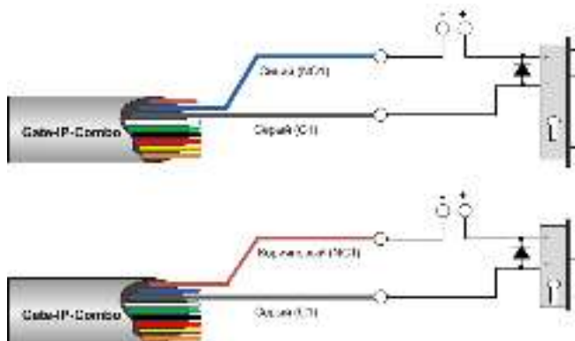
Рис.19. Подключение замков
