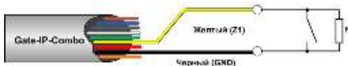
Рис.15. Подключение кнопки запроса прохода
