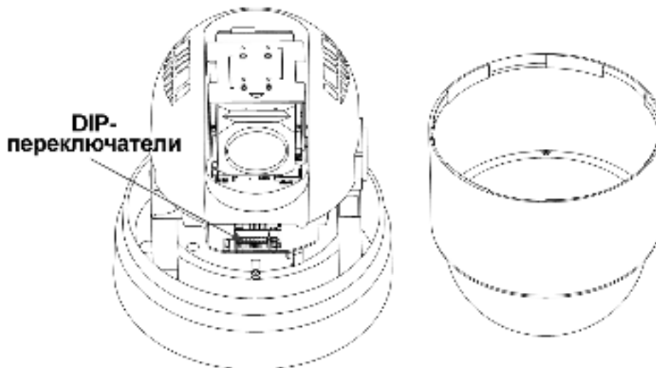
Рис. 1.2. Расположение DIP-переключателей
