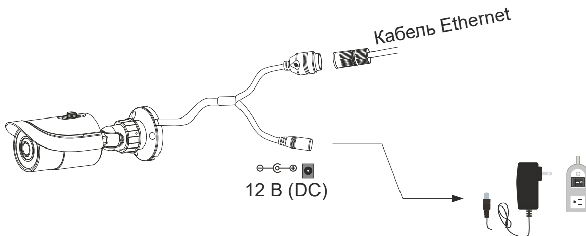
Рис. 3.2. Подключение кабелей
