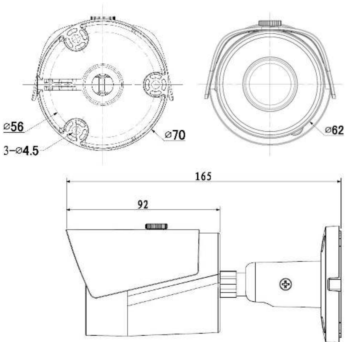
Рис. 1 Размеры камеры
