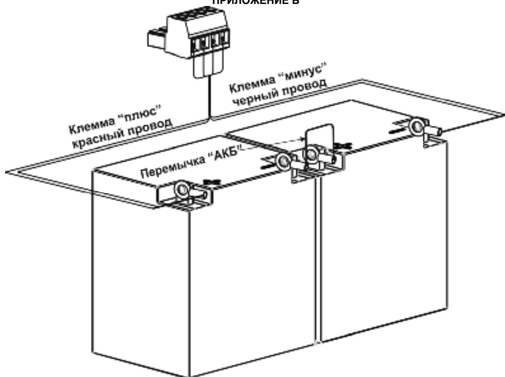
Схема соединения аккумуляторов в батарею
