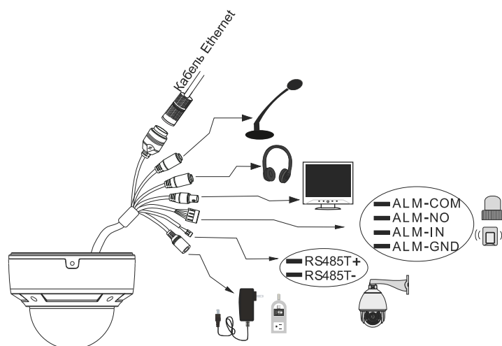
Рис. 3.2. Подключение кабелей
