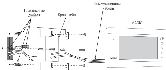
Рис. 4 Монтаж видеодомофона
