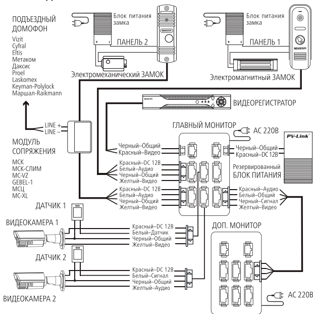
Рис. 7 Схема подключения видеодомофонов MAGIC HD
