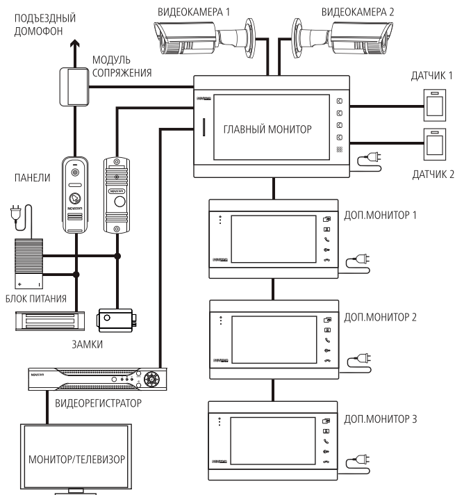
Рис. 6 Функциональная схема системы на базе видеодомофонов MAGIC HD
