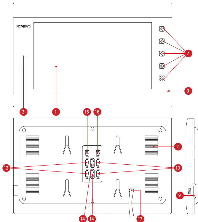
Рис. 3 Описание видеодомофона MAGIC 10 HD
