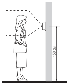
Рис. 5 Рекомендуемая высота установки видеодомофона
