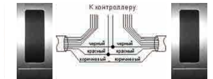
Рисунок 3 – Подключение синхронизированных считывателей
