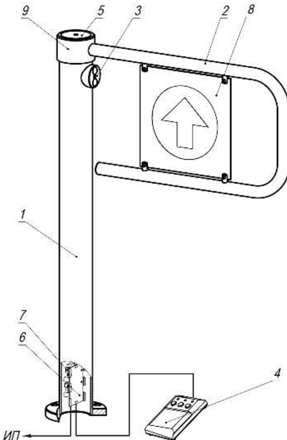
1 – стойка калитки, 2 – створка калитки, 3 – МИ, 4 – ПДУ с кабелем (контроллер СКУД 1 /устройство РУ 1 ), 5 – крышка, 6 – кронштейн, 7 – МК, 8 – заполнение створки с комплектом держателей, 9 – узел вращения.
