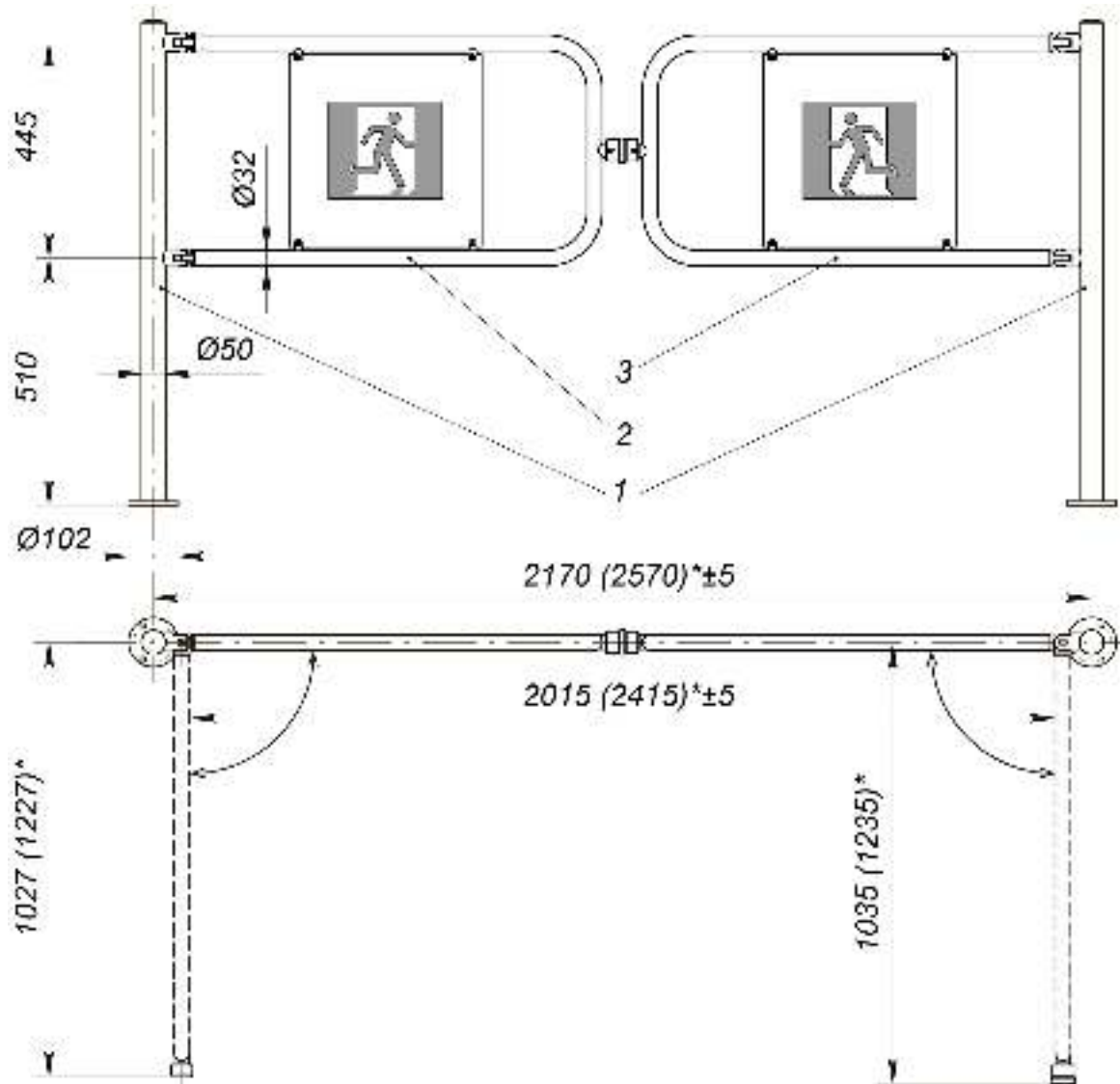
Рисунок 7. Двойная распашная секция ограждения с магнитным УБ 1 : 1 – стойка BH02 2-00(01,02,03); 2 – створка BH02 1-18(19) с магнитным УБ; 3 – створка BH02 1-18(19) с ответной частью магнитного УБ
