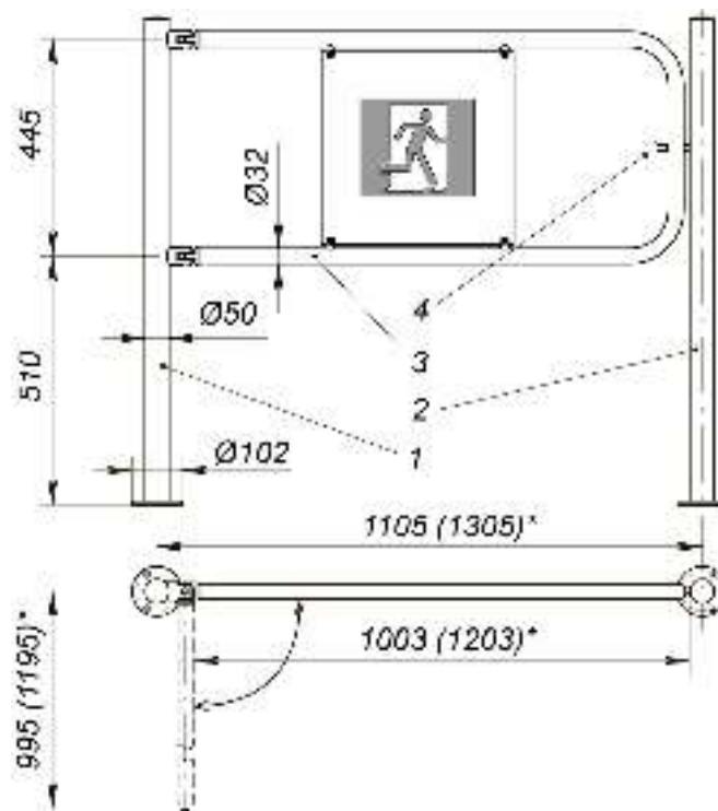
Рисунок 5. Поворотная секция ограждения с механическим УБ 1 : 1 – стойка ВН02 2-00(01,02,03); 2 – стойка ВН02 2-14(15,16) с отверстием для мех. УБ; 3 – створка ВН02 1-16(17) с механическим УБ; 4 – ручка механического УБ
