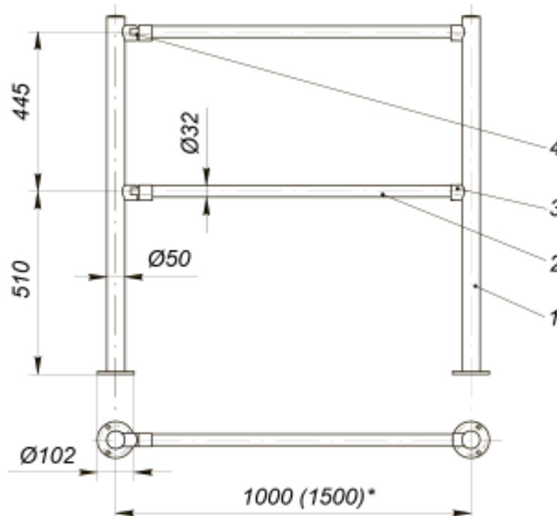
Рисунок 4. Секция ограждения без заполнения с поворотными патрубками 1 : 1 – стойка BH02 2-00(01,02,03); 2 – поручень BH02 1-00(01); 3 – патрубок BH02 0-10; 4 – патрубок поворотный BH02 0-11
