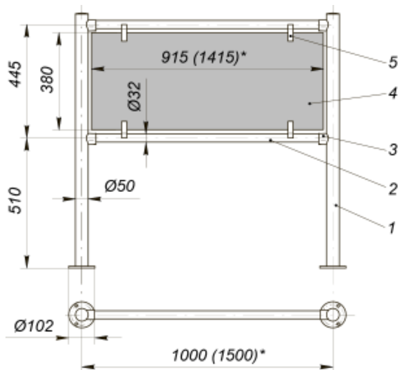
Рисунок 1. Стационарная секция ограждения с заполнением 1 : 1 – стойка ВН02 2-00(01,02,03); 2 – поручень ВН02 1-00(01); 3 – патрубок ВН02 0-10; 4 – заполнение (стекло или полимерный материал); 5 – держатель ВН02 0-02
