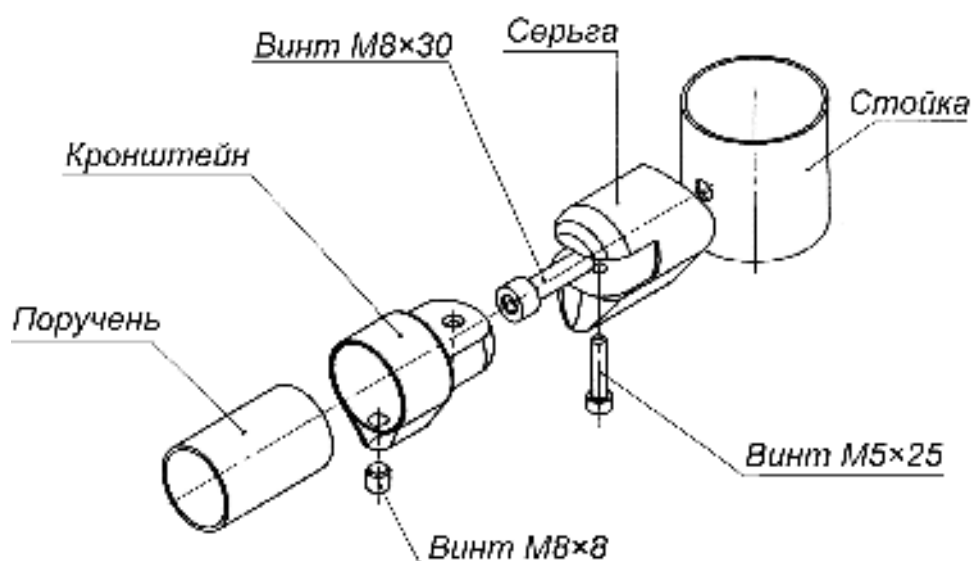
Рисунок 10. Схема крепления поручней к стойкам ограждения с использованием поворотного патрубка BH02 0-11
