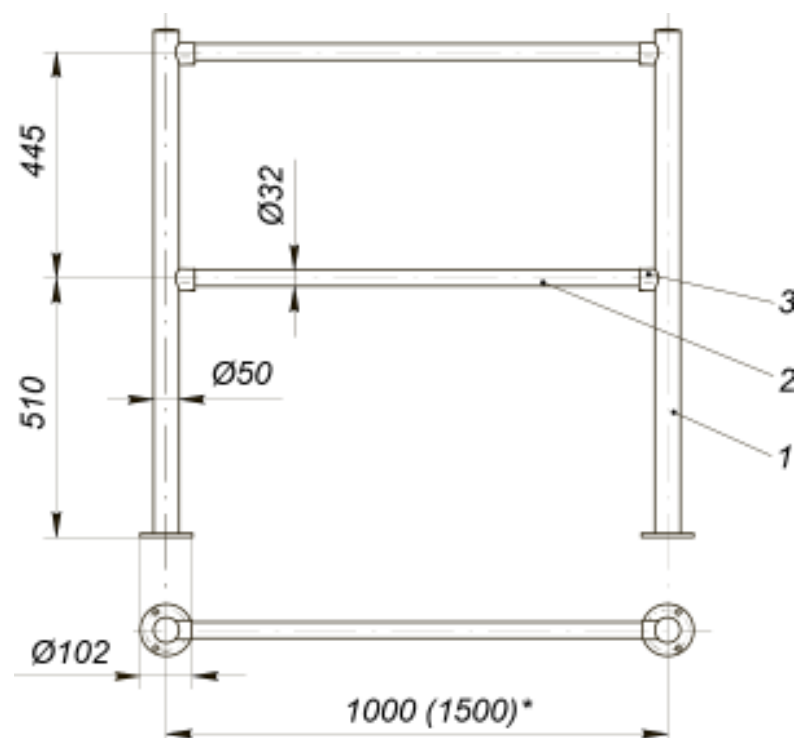
Рисунок 2. Стационарная секция ограждения без заполнения 1 : 1 – стойка ВН02 2-00(01,02,03); 2 – поручень ВН02 1-00(01); 3 – патрубок ВН02 0-10
