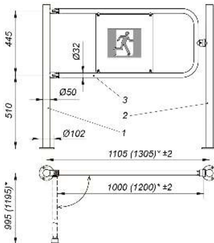
Рисунок 6. Автоматическая поворотная секция ограждения с электромагнитным УБ 2 : 1 – стойка ВН02 2-00(01,02,03); 2 – стойка ВН02 2-04(05,06)/EL с электромагнитным УБ; 3 – створка ВН02 1-06(07)/EL
