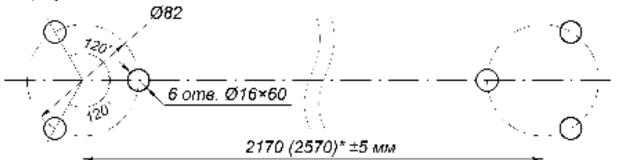
Рисунок 17. Схема разметки отверстий для установки фланцев двойной распашной секции ограждения с магнитным УБ
