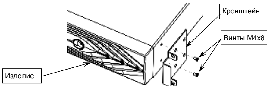
Рисунок 4 — Установка кронштейнов на корпус изделия
