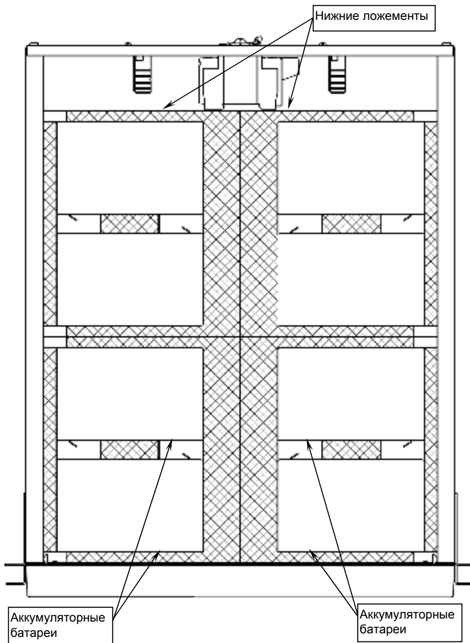
Рисунок 3 – Размещение аккумуляторных батарей в корпусе.
