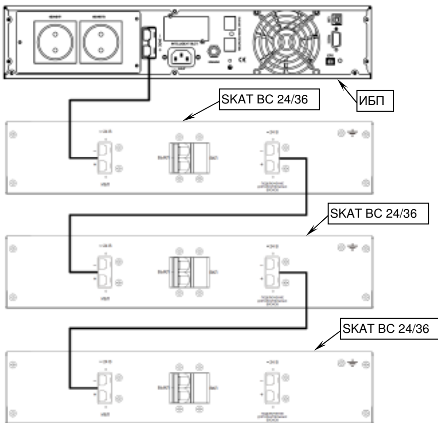
Рисунок 5 — Подключение ИБП и дополнительных батарейных блоков
