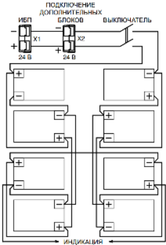
Рисунок 7 — Схема соединений аккумуляторных батарей
