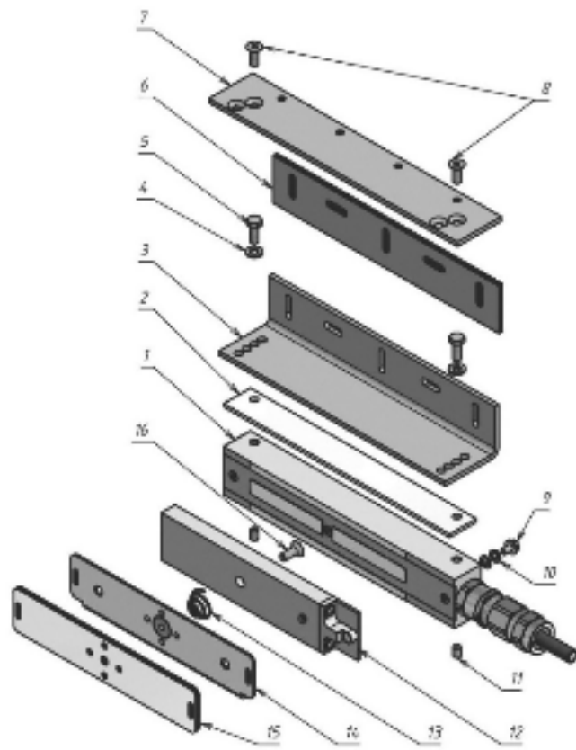
Рисунок 1- Комплект поставки
