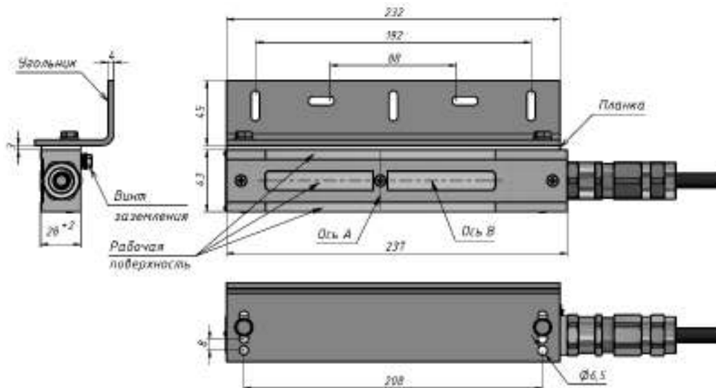
Рисунок 6 - Корпусная часть
