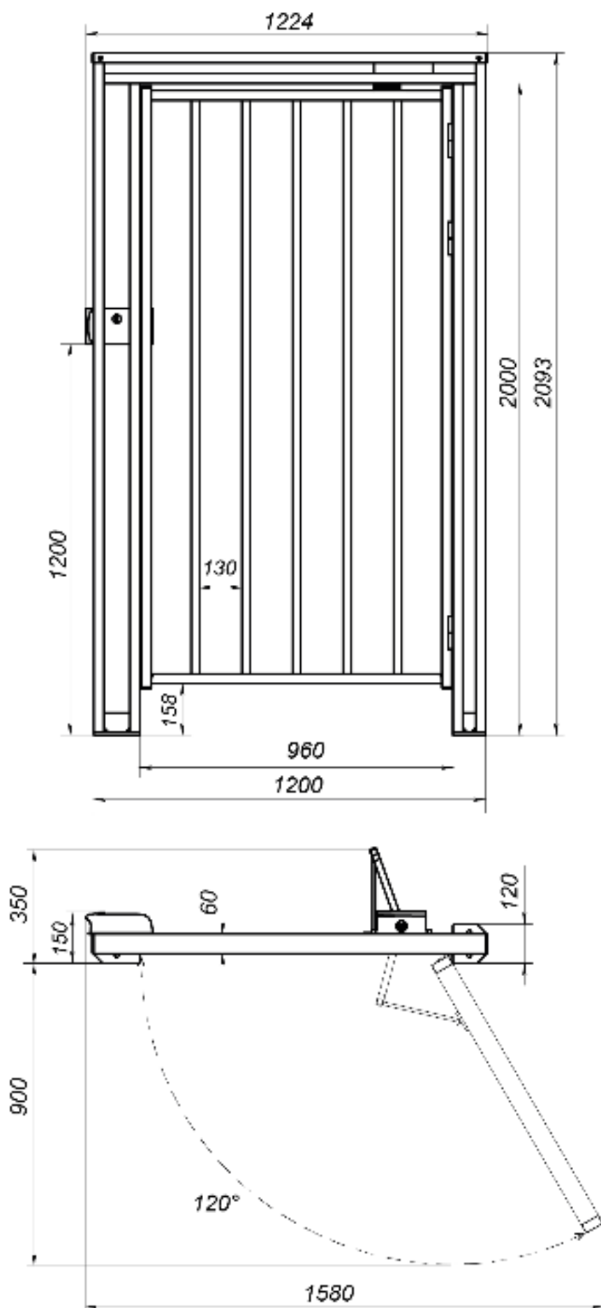
Рисунок 2. Габаритные и промежуточные размеры
