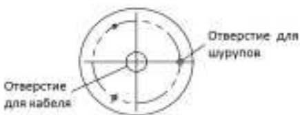
Рисунок 2-9 Шаблон крепления
