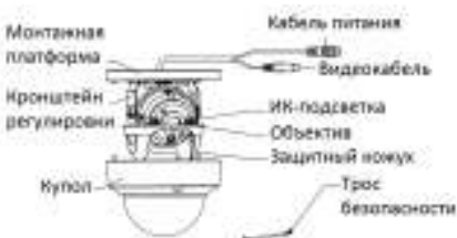
Рисунок 1-3 Камера III типа
