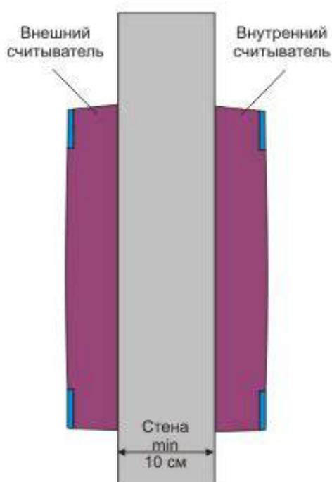
Рисунок 4. Крепление считывателей на одном уровне.
