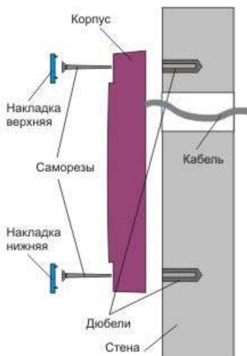
Рисунок 3. Крепление считывателя PR-EH09.
