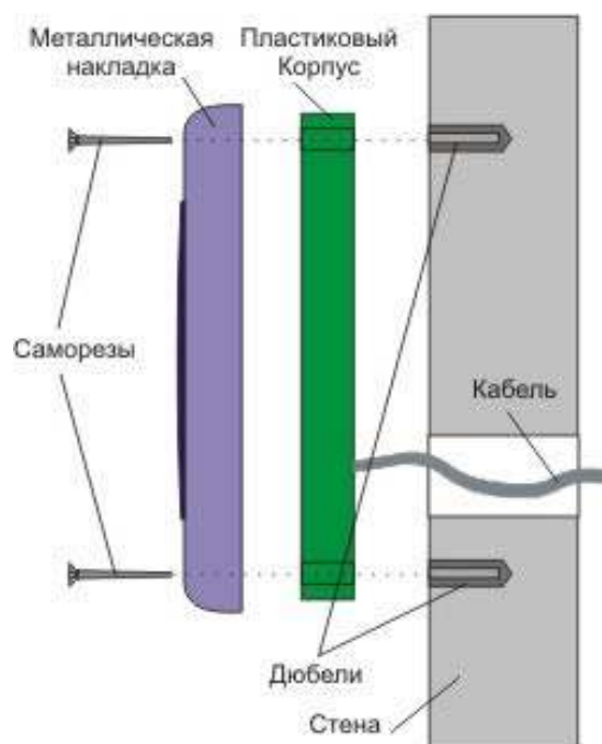
Рисунок 2. Крепление считывателя PR-EH05.
