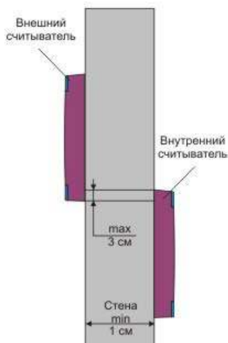
Рисунок 5. Крепление считывателей с разнесением по вертикали.
