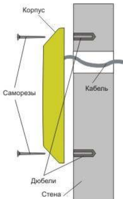
Рисунок 1. Крепление считывателя PR-EH03.
