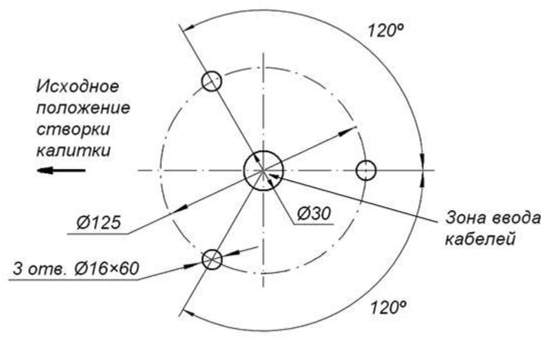
Рисунок 9. Схема разметки для монтажа калитки
