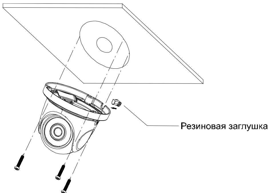
Рис. 5.2. Крепление видеокамеры
