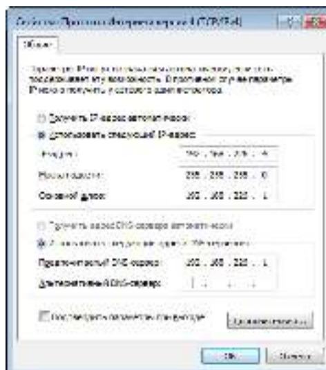
Рис. 6.6. Настройки IP-протокола
