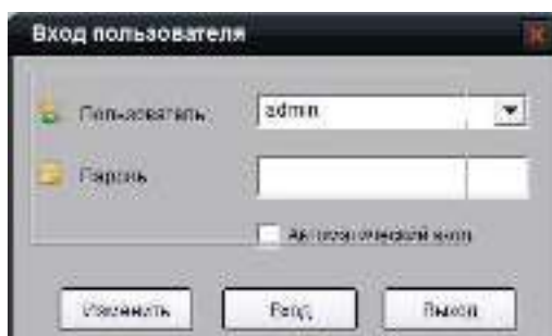
Рисунок 4.2.2 Авторизация пользователя
