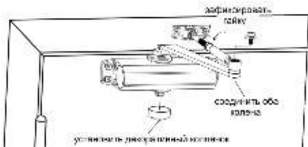
Рисунок 2 – Вариант вертикальной установки
