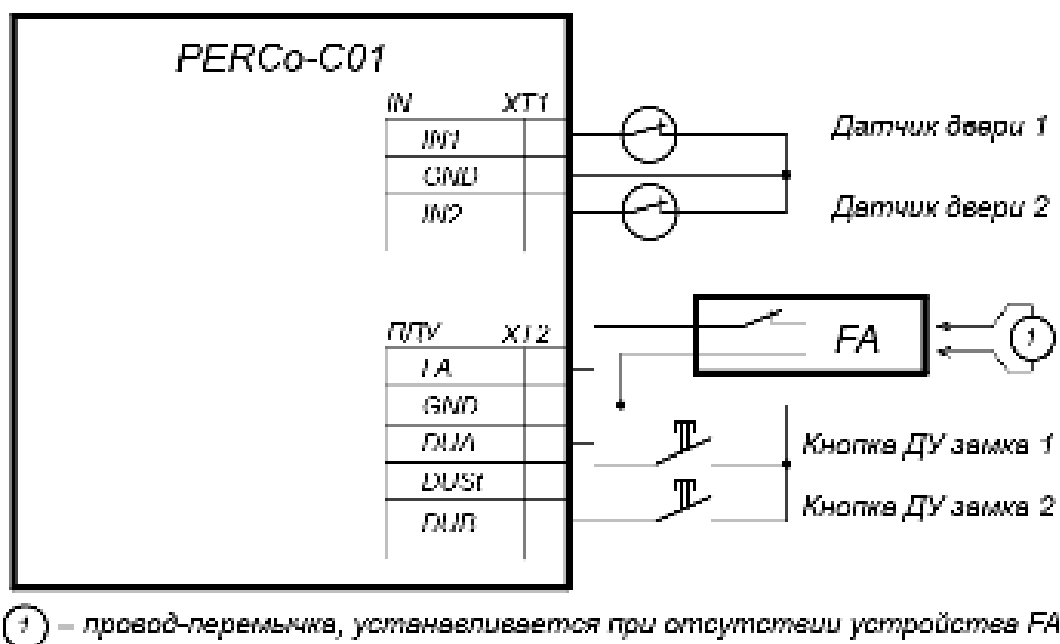
Рисунок 8. Схема подключений кнопок ДУ и датчиков двери
