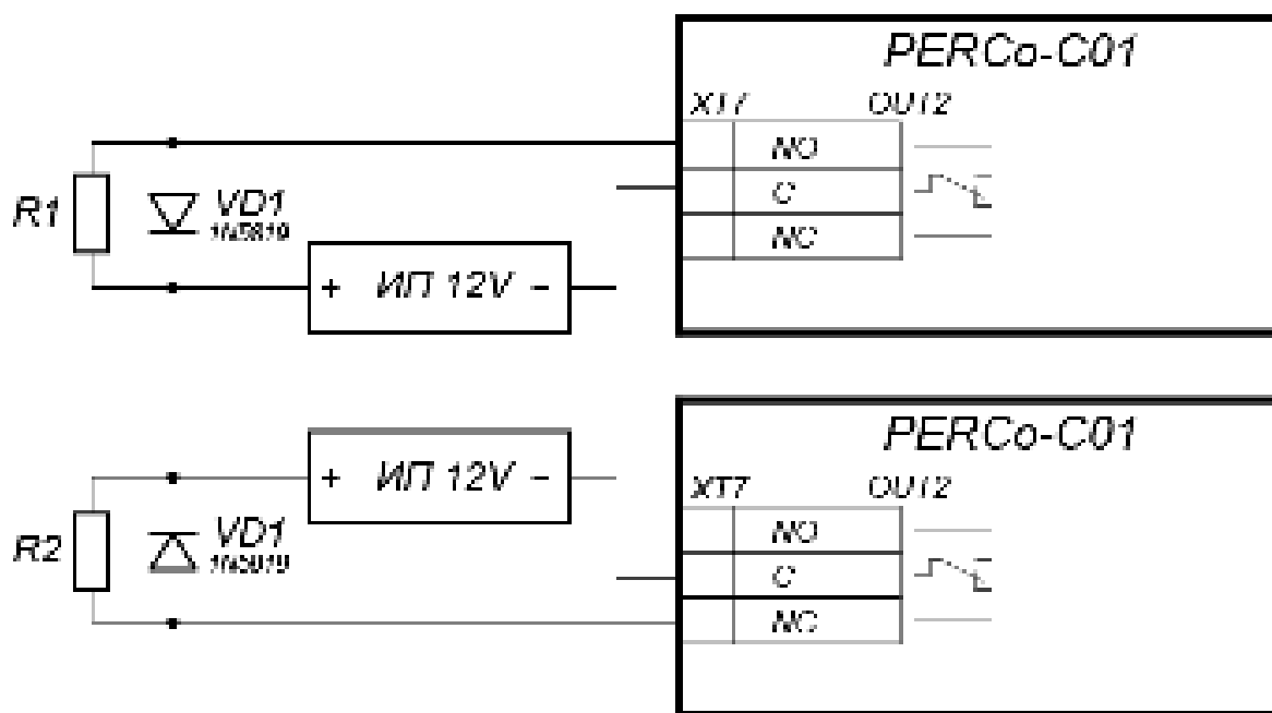
Примеры подключения
