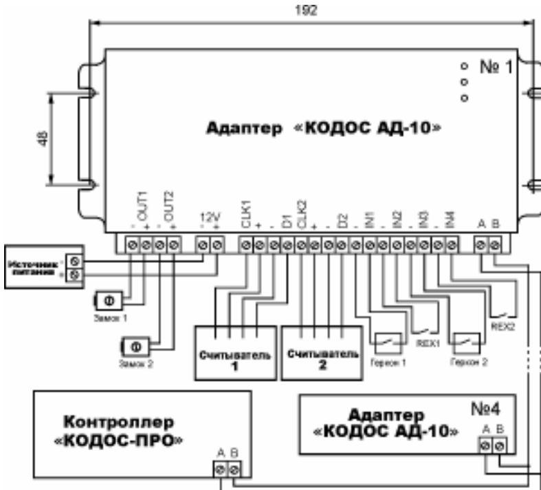
Рисунок 2 – Схема подключения адаптера
