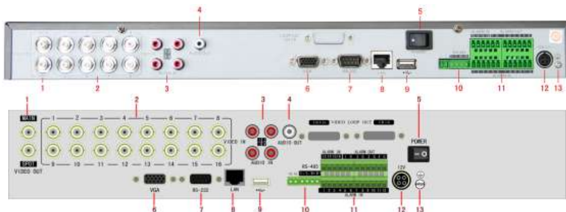
Рис 8. Задняя панель цифрового регистратора
