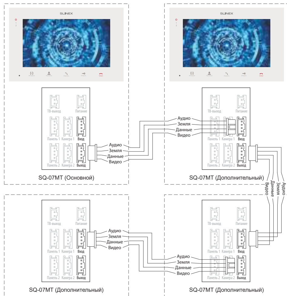
Схема 2. Подключение системы домофонов SQ-07MT.
