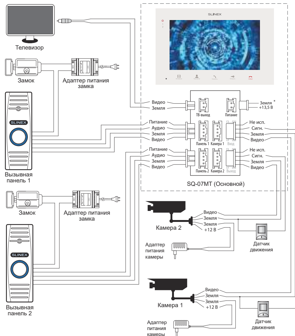
Схема 1. Подключение вызывных панелей, камер и телевизора к домофону SQ-07MT
