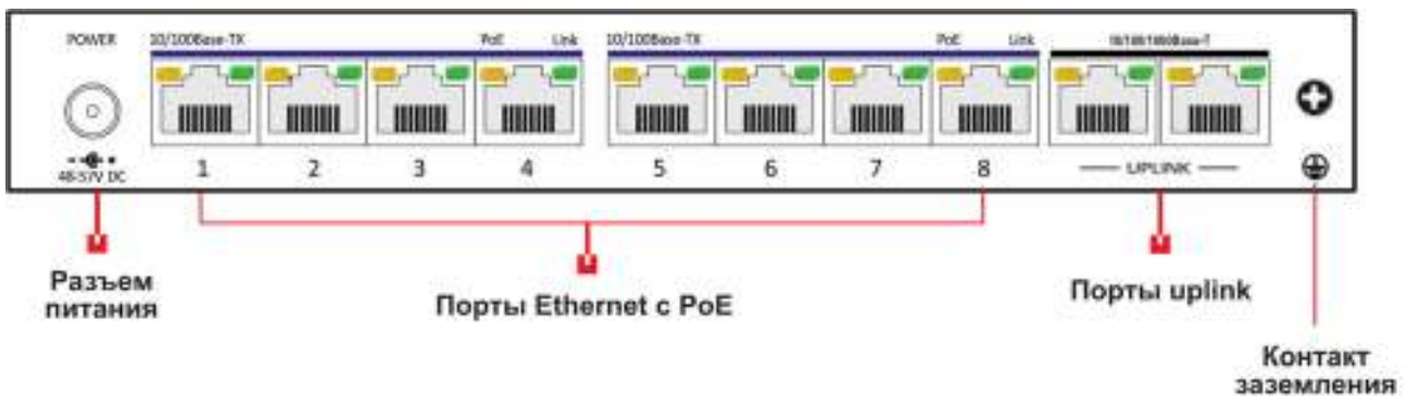
Рис. 2.2. Задняя панель
