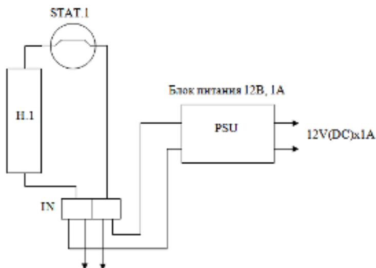
Рис.2.1. Принципиальная электрическая схема подключения LTV-HEM-300H-12-220 и LTV-HEB-300H-12-220
