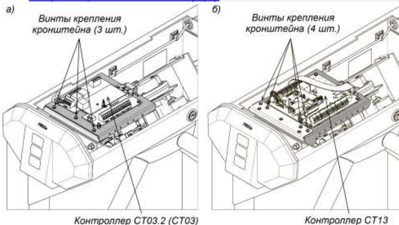
Рисунок 1. Крепление кронштейна контроллера ЭП
