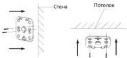
Рисунок 2-4 Установка монтажной платформы
