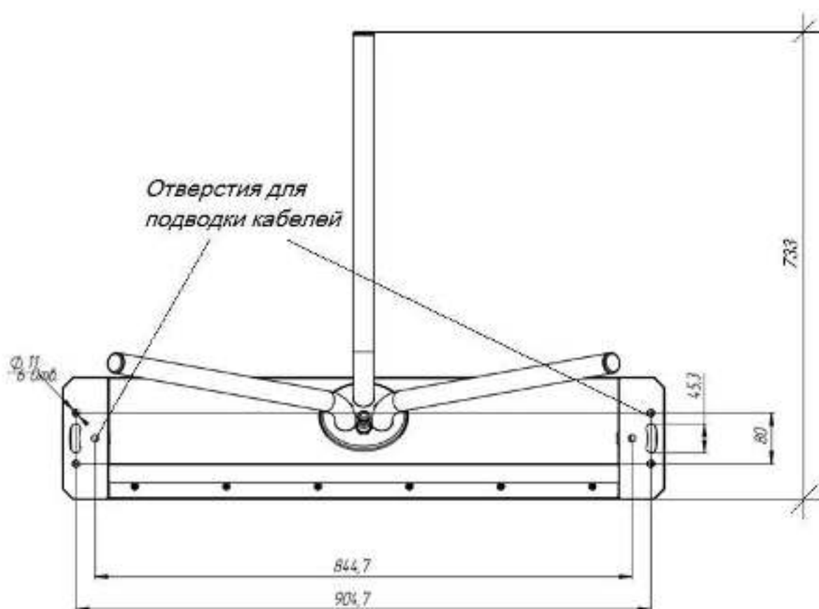
Рис. 11. . Установочные размеры
