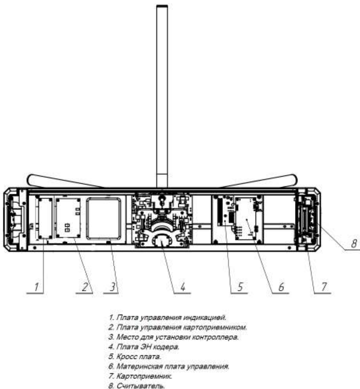
Рис. 13. Расположение плат в стойке турникета
