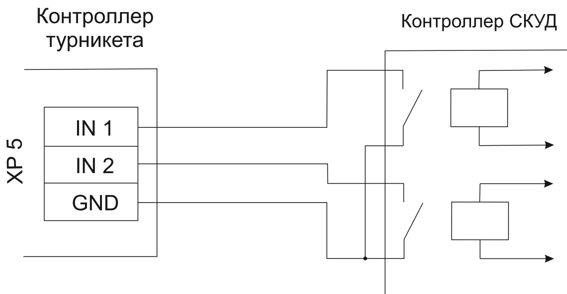
Рисунок 8.2.2 Схема подключения турникета к стороннему СКУД
