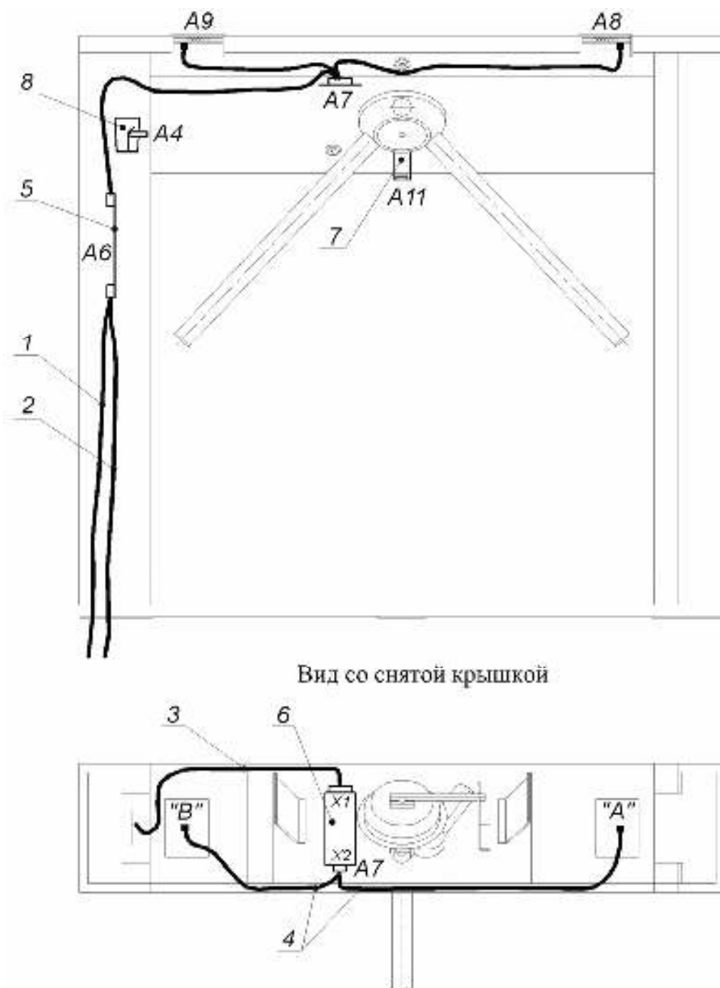
Рисунок 11. Схема прокладки кабелей в стойке турникета:
