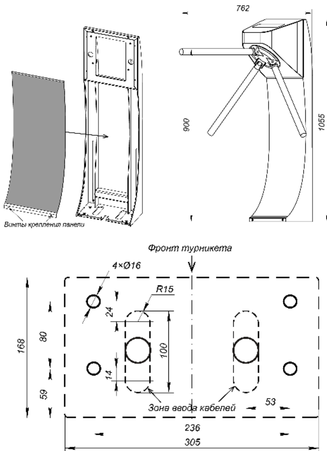
Рисунок 16. Внешний вид и схема разметки отверстий для монтажной стойки PERCo-MT10.3
