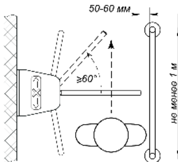
Рисунок 13. Рекомендации по организации зоны прохода
