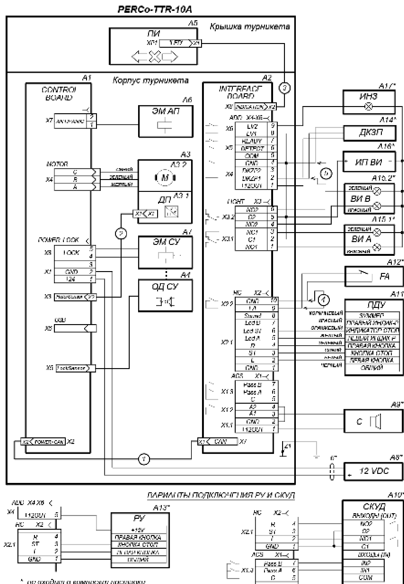
Рисунок 17. Схема электрическая соединений
