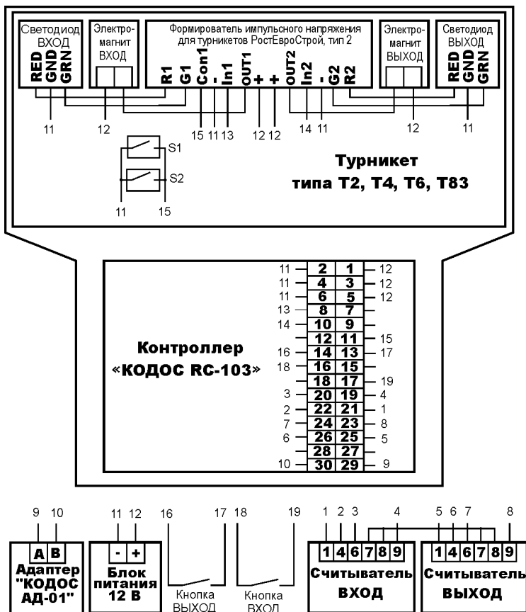
Рисунок 14 – Блок-схема подключения турникетов компании «РостЕвроСтрой» серии Т2, Т4, Т6, Т83 с формирователем импульсного напряжения тип 2
