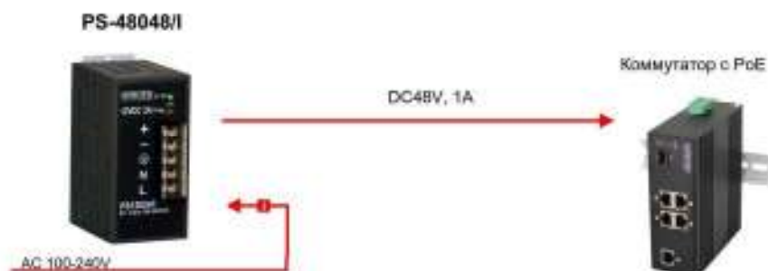
Рис. 5 Подключение PS-48048/I
