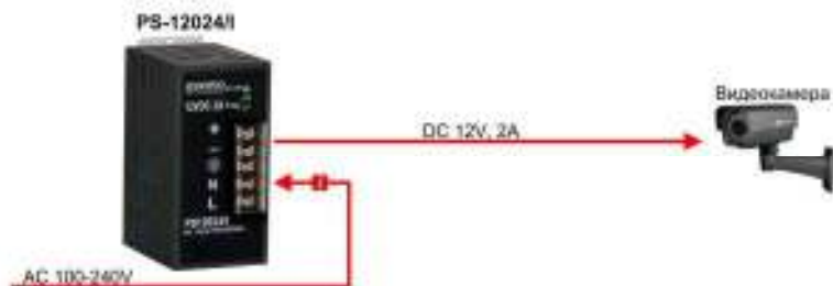
Рис. 4 Подключение PS-12024/I
