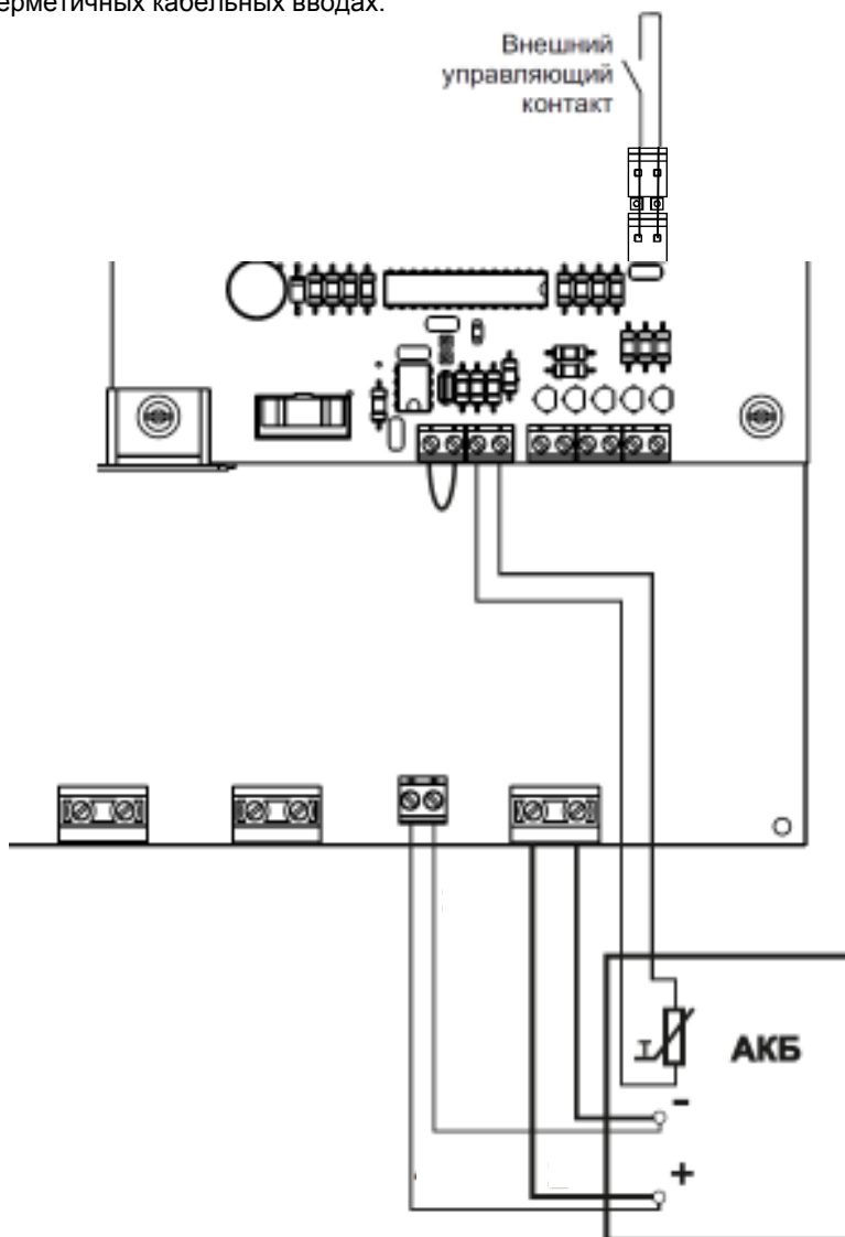
Рисунок 5 – Подключение АКБ, термодатчика и внешнего контакта
