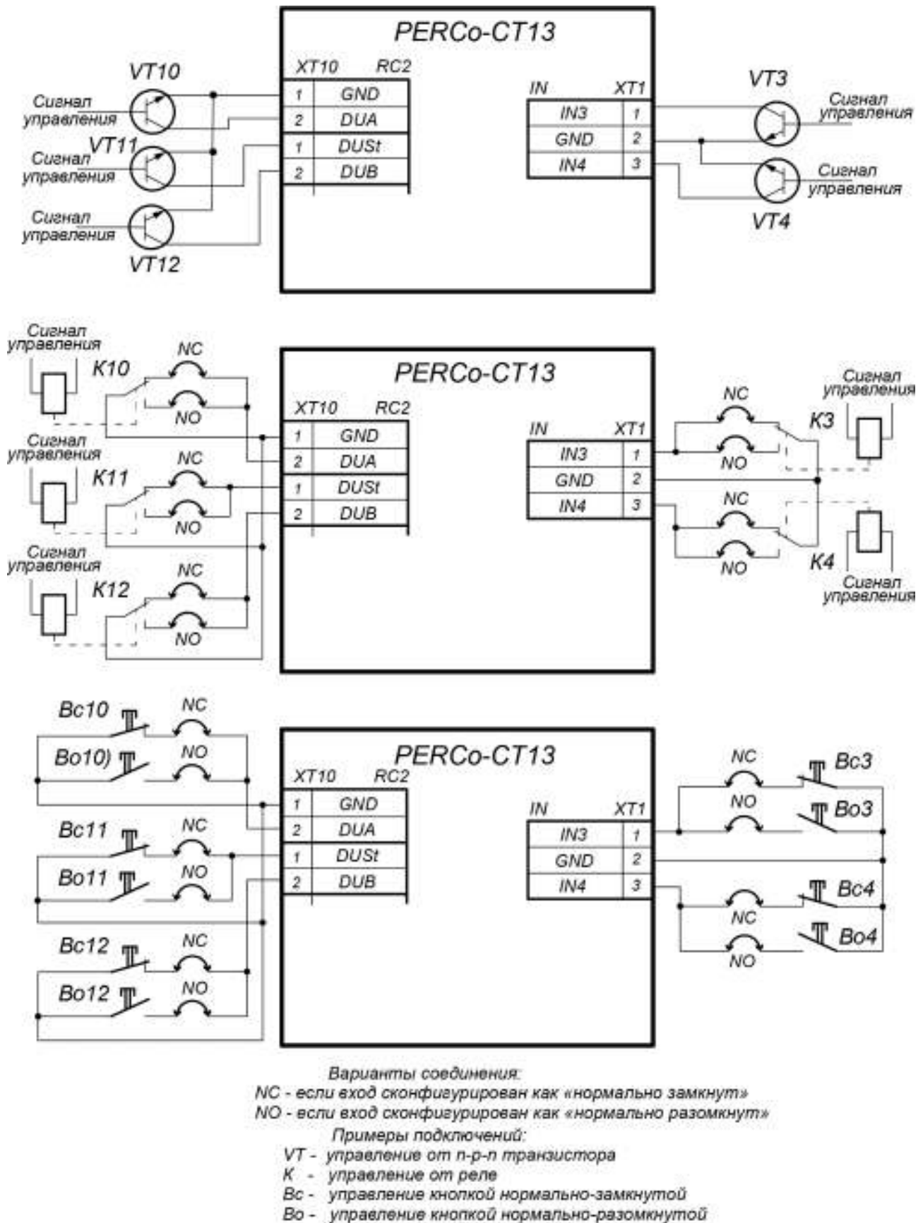
Рисунок 23. Схема подключений доп. оборудования к входам контроллера
