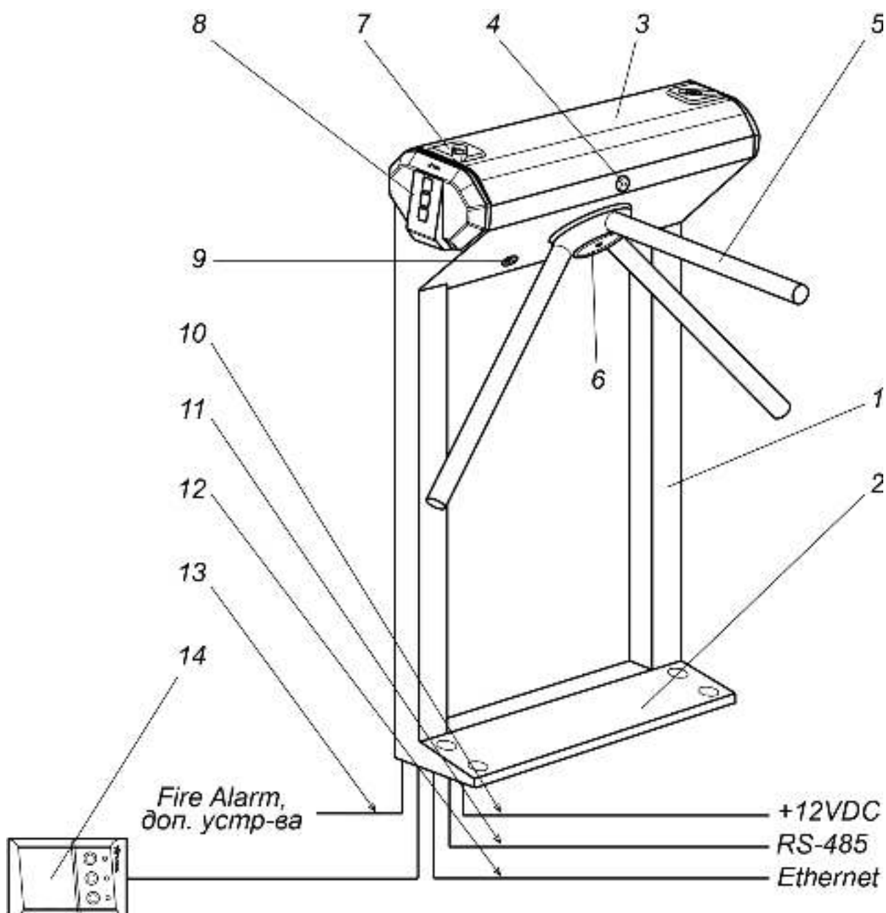
Рисунок 2. Устройство ЭП
